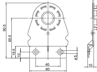
Befestigungswinkel 6482
