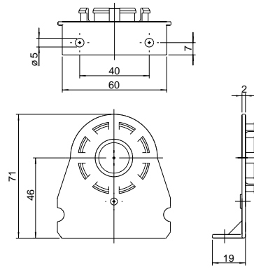
Befestigungswinkel 6482
