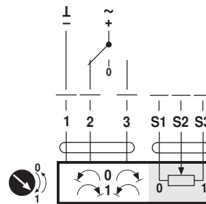
AC/DC 24 V, 3-punts
